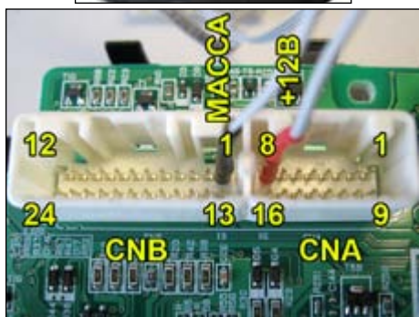
Питание CNB1: масса; CNA8: +12В
