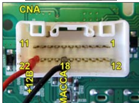
Питание 18: масса; 22: +12В
