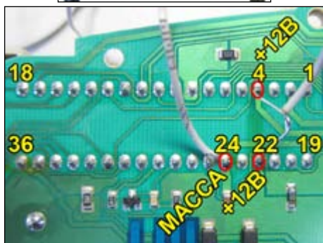
Питание 24: масса; 4 и 22: +12В
