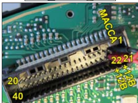
Питание 1: масса; 21 и 22: +12В
