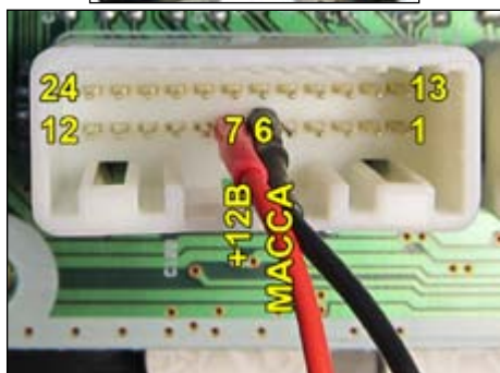
Питание 6: масса; 7: +12В
