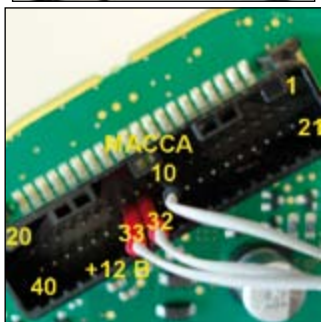
Питание 10: масса; 32 и 33: +12В
